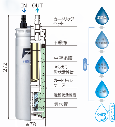
クイックジョイントにワンタッチで接続し、ロック用保護カバーでカートリッジが外れないようロックすることで、簡単にカートリッジの交換ができます。
